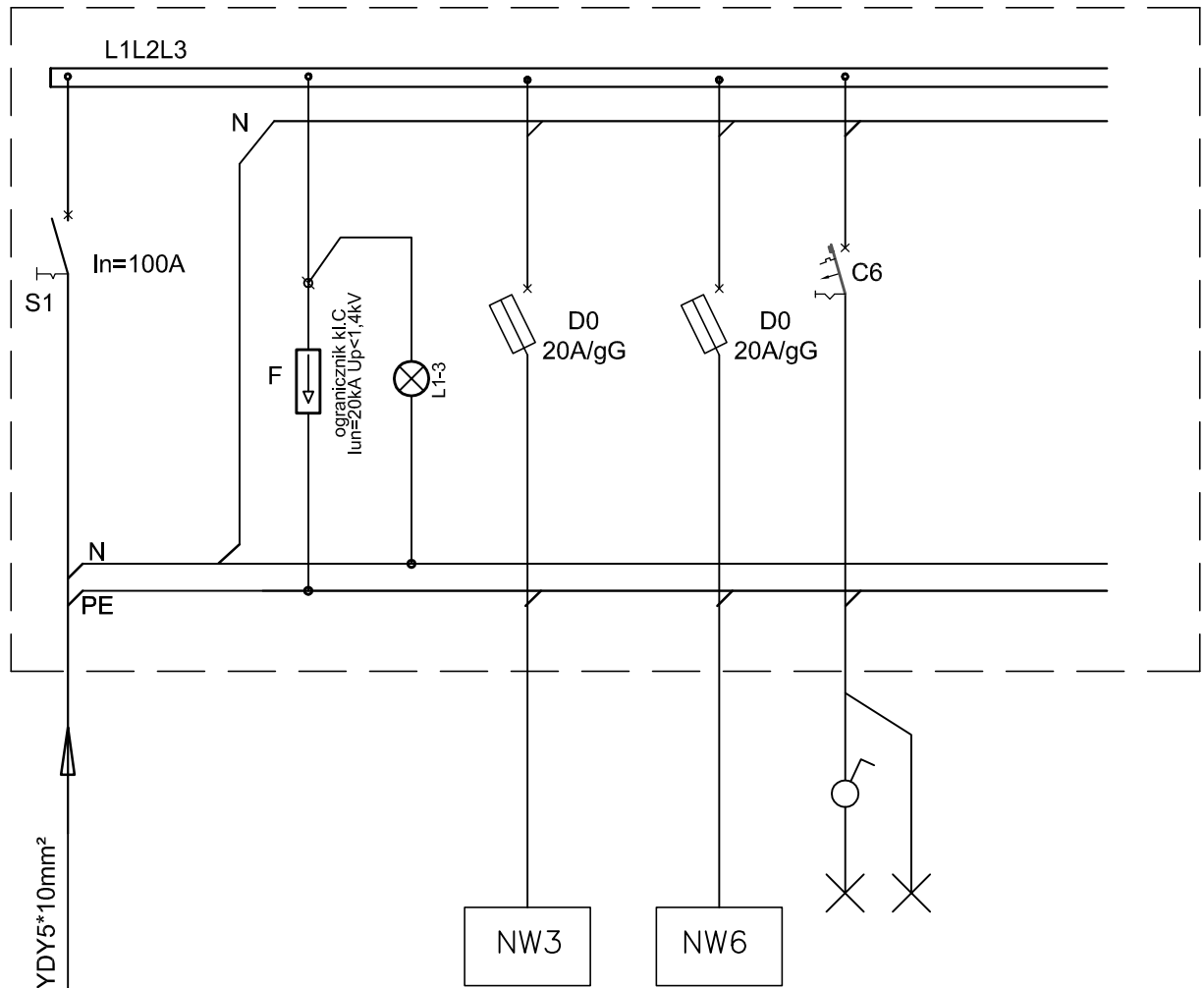
TABLICA ROZDZIELCZA WENTYLACJI Tw2
