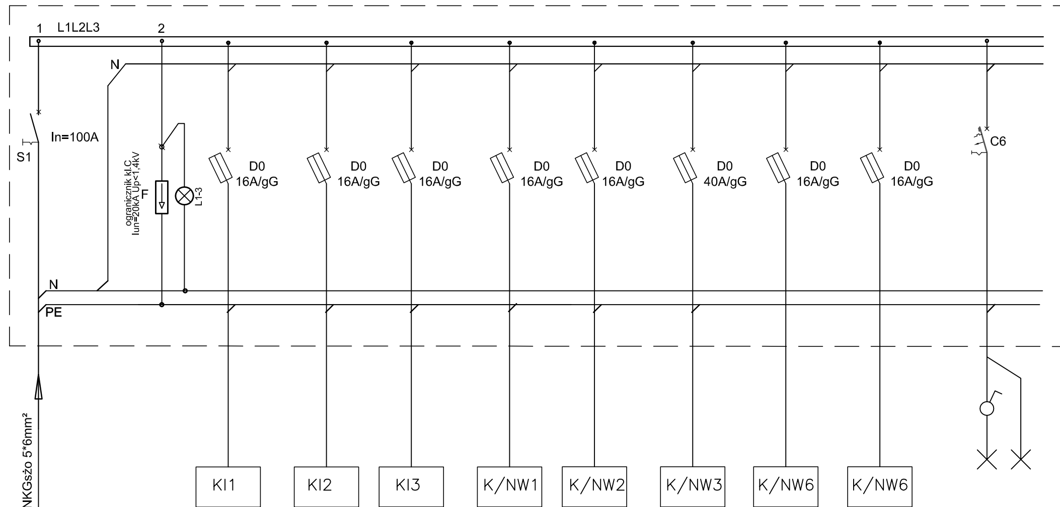
TABLICA ROZDZIELCZA WENTYLACJI Tki
